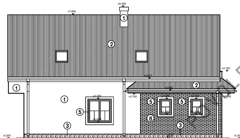
POHLAD BOČNÝ
