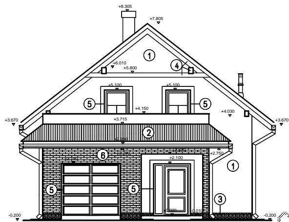
POHLAD ČELNÝ
